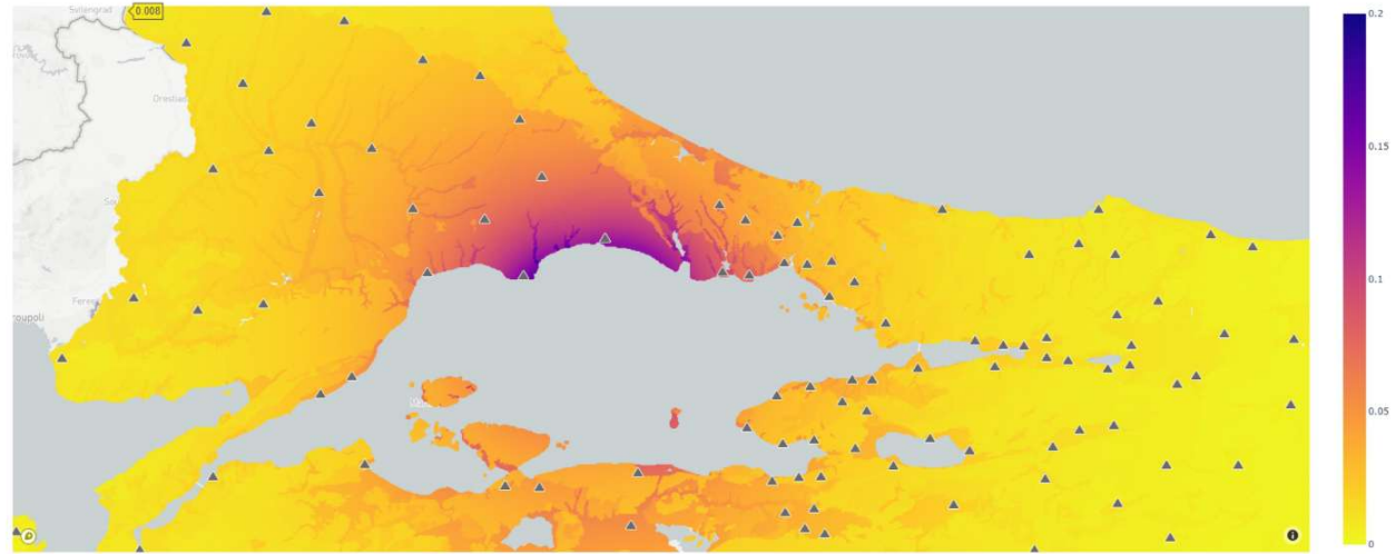
Şekil 8. Farklı azalım ilişkileri formulleri ile Mw 6.2 lik depremi ivme dağılımları modelleme MATAM Bu haritalarda siyah üçgenler ölçüm noktalarını gösterir. Şekil 7 de bu noktalar ile haritada hesaplanan değerleri karşılaştırması bulunmaktadır. Azalım ilişkileri ile yapılan MATAM veri tabanı kullanılarak yapılan taban haritaları üzerinde yapılan hesaplamalarda formüllerin dayandığı
